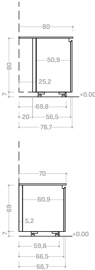
Modulo base con sistema Organizer / Giorno Base module with Organizer system / Open unit
