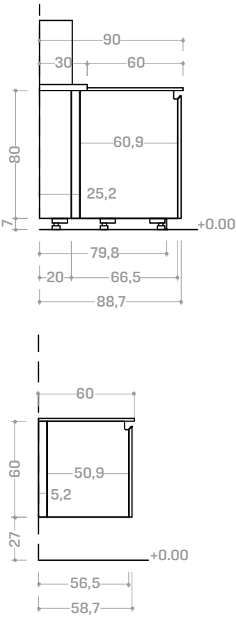
Modulo base con scaffale Medley tipo A-B Base module with Medley type A-B shelf
